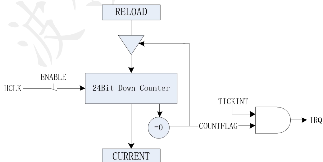
图 5-4-1 Systick 模块结构图
