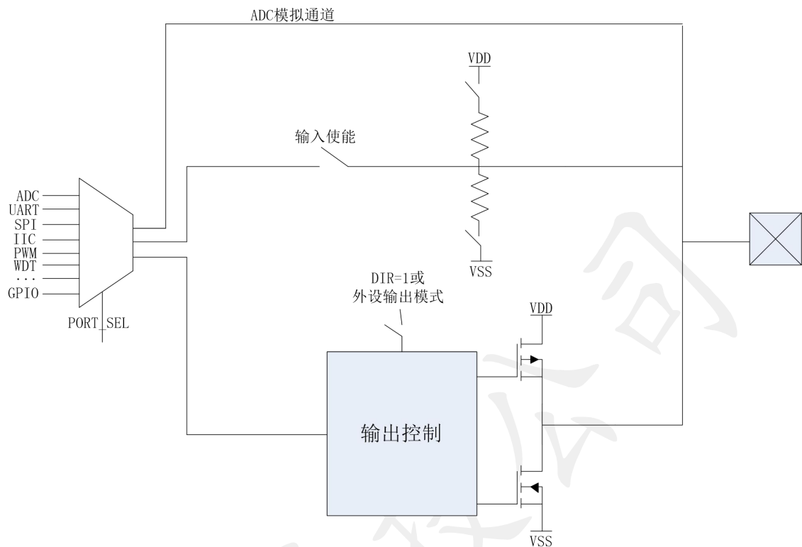
图 5.8.1 PORTCON 模块结构框图
